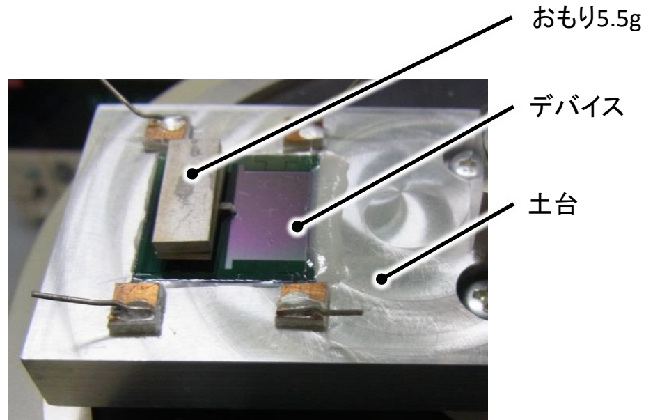
パッケージ外観
