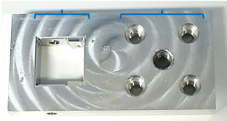
アルミ土台
